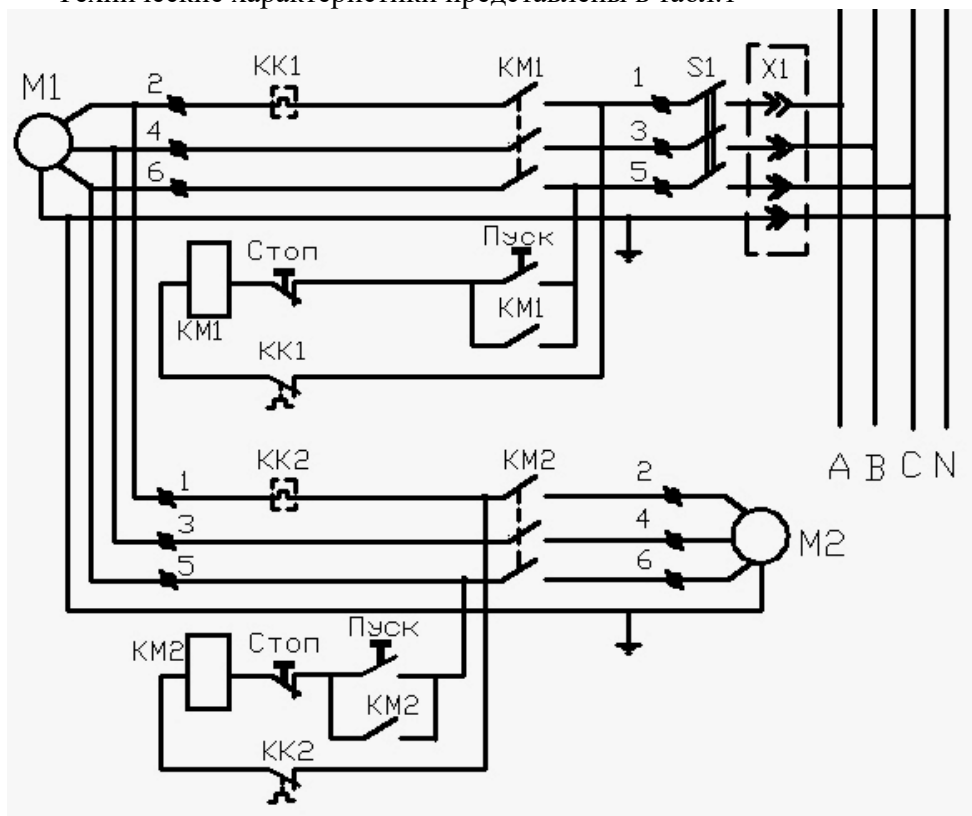
Рис. 2 Принципиальная электрическая схема станка ПСР-А.
