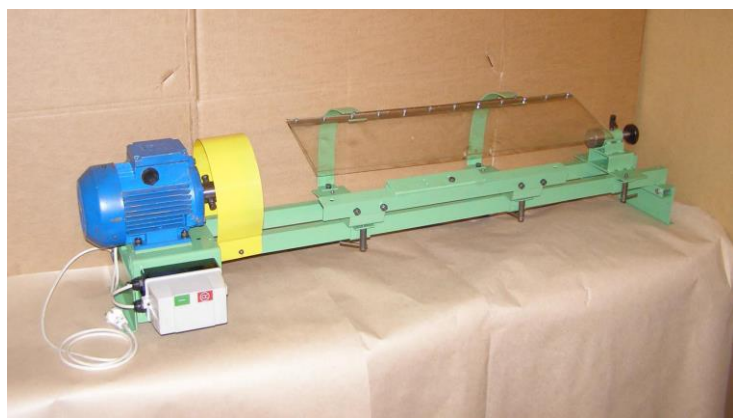
Токарный станок ДОС-Т1000У (настольное исполнение)
